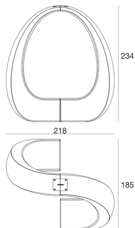
Arche · 218 × 185 × 234 cm
