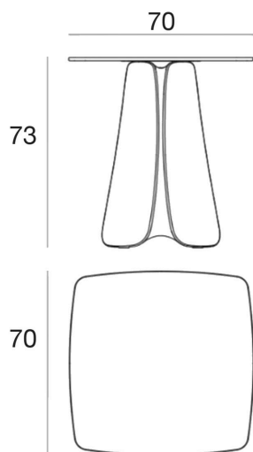
70 × 70 × 73 cm
